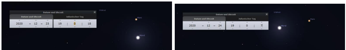
Abbildung 4: Der Anblick des Himmels am 23. und 24. Dezember 2020 gegen 8 Uhr. (Bild: www.stellarium.com)
