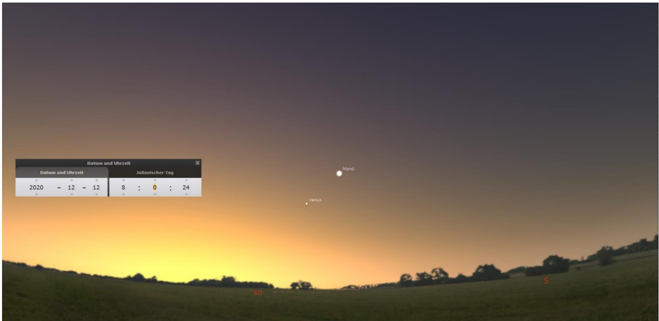
Abbildung 1: www.stellarium.com
