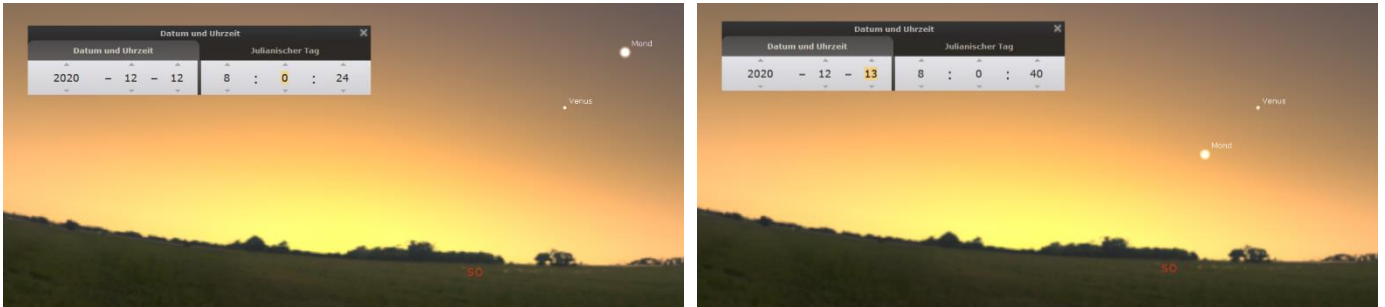
Abbildung 2: Der Anblick des Himmels am 12. und 13. Dezember 2020 gegen 8 Uhr. (Bild: www.stellarium.com)
