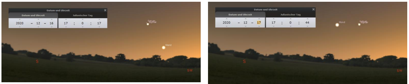
Abbildung 3: Der Anblick des Himmels am 16. und 17. Dezember 2020 gegen 17 Uhr. (Bild: www.stellarium.com)
